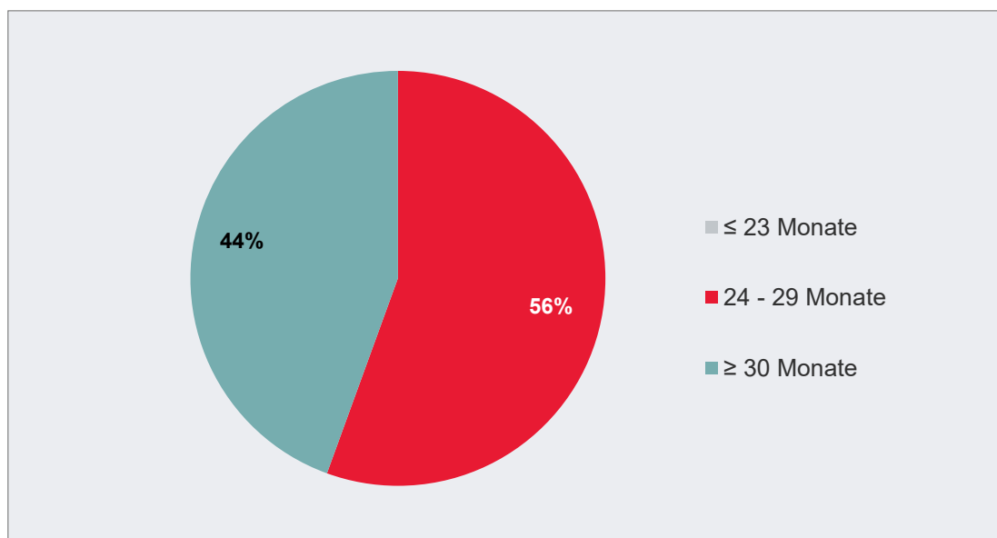
Abbildung 2-4: Netzwerklaufzeiten (n=72)
